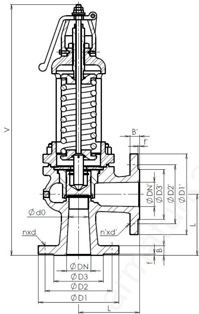
Hlavní a připojovací rozměry PN 40/16 (vstup/výstup)
